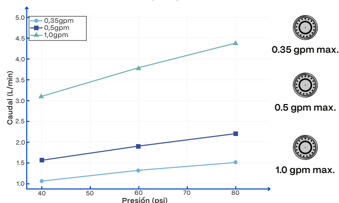
Caudal vs Presión por tipo de aireador
