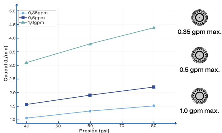
Caudal vs Presión por tipo de aireador
